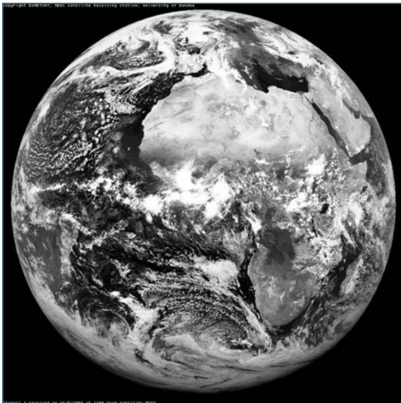
Abb. 2: Die Wolkenbänder und Luftwirbel auf dem Satellitenbild lassen die komplizierten Windsysteme auf der Erde erahnen.
